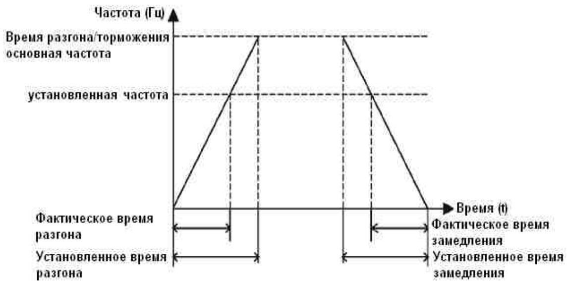
Рисунок 6-1 Время разгона/торможения
