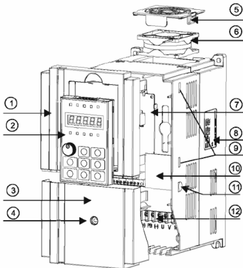
Рисунок 2-1 Принципиальная схема структуры преобразователя частоты
