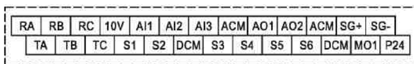
рисунок 3-4. Клеммы управления преобразователя частоты
